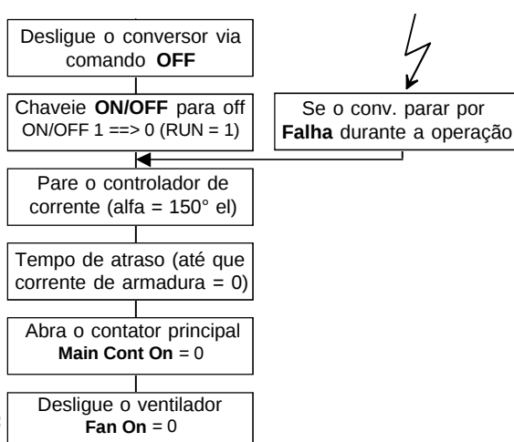
Fig. 4.4/2: Seqüência para desligar o DCS 400
