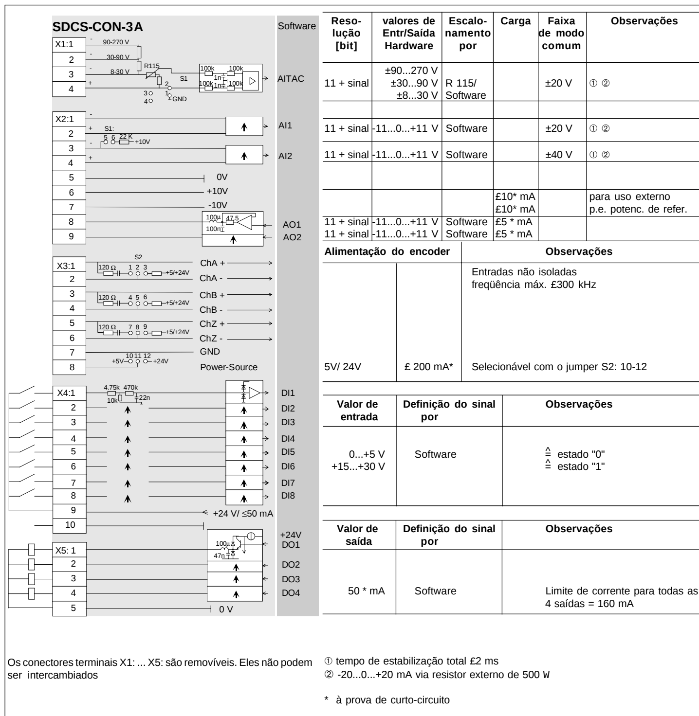
Fig. 3.5/3 Conexão terminal do cartão SDCS-CON-3A
