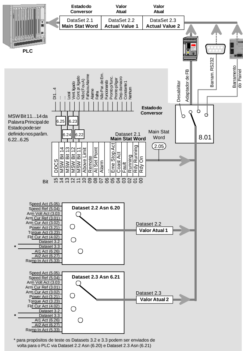
Fig.: 7/2 Visão geral do Dataset 2. Monitorando o conversor via comunicação fieldbus
