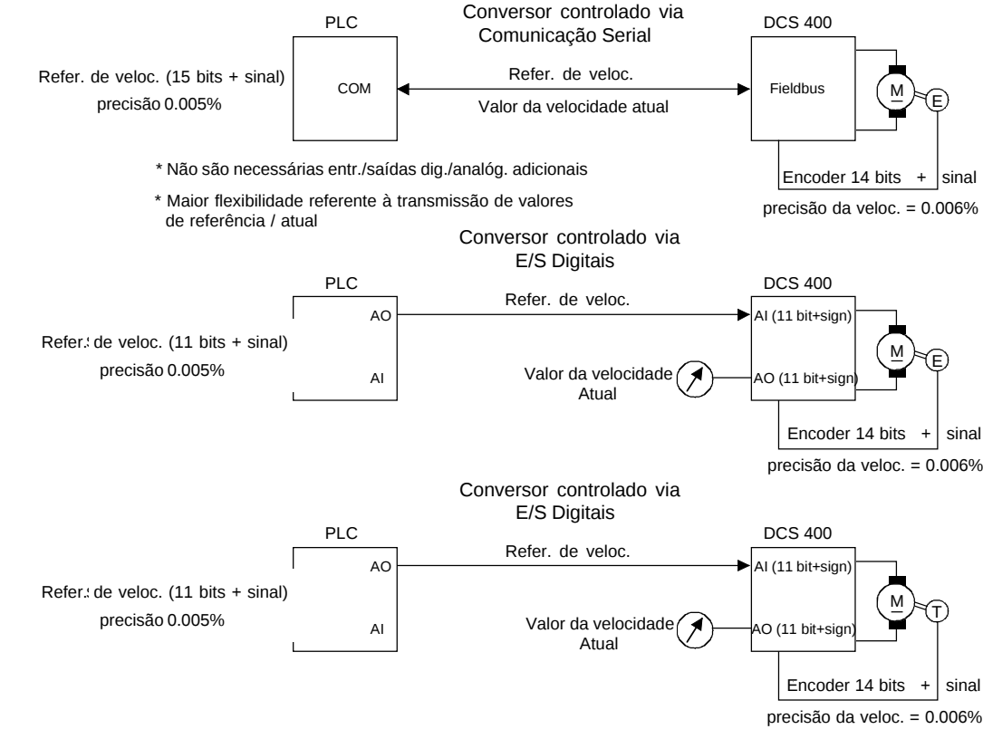
Fig. 4.3/1: Comparação da precisão entre os diferentes modos de controle
