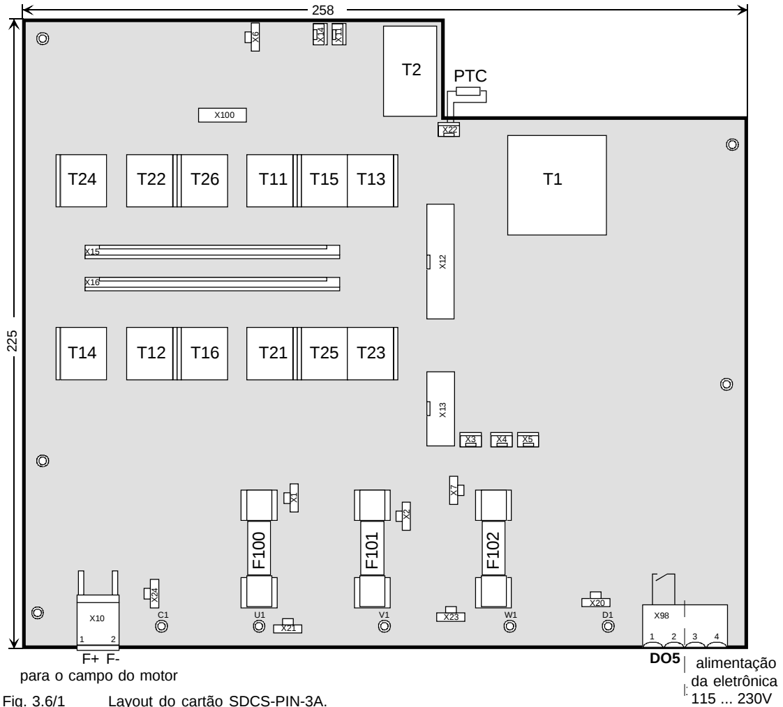
Fig. 3.6/1 Layout do cartão SDCS-PIN-3A.
