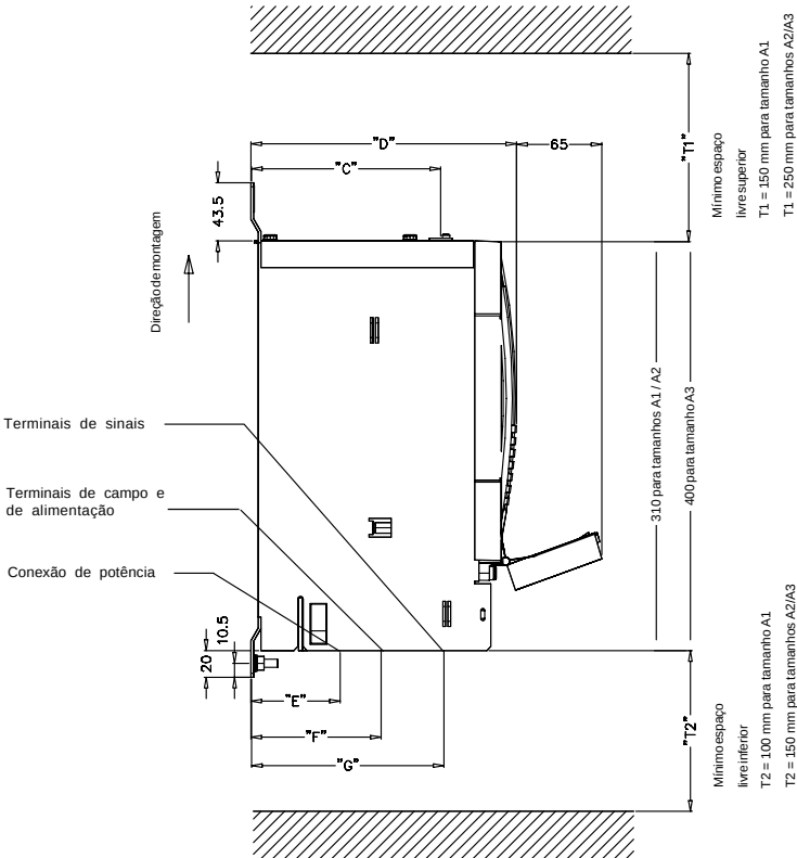
Fig. 3.1/1: Desenho dimensional dos módulos A1, A2, A3
