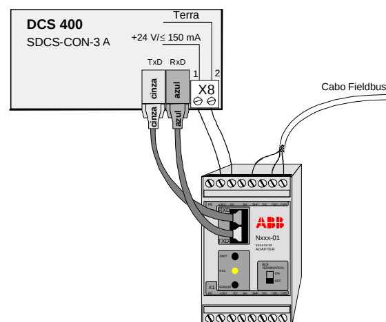
Fig.: 7.3/2 Conexão do Adaptador de Fieldbus para o DCS 400
